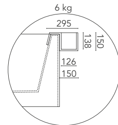
Contenitore / Behälter / Container
